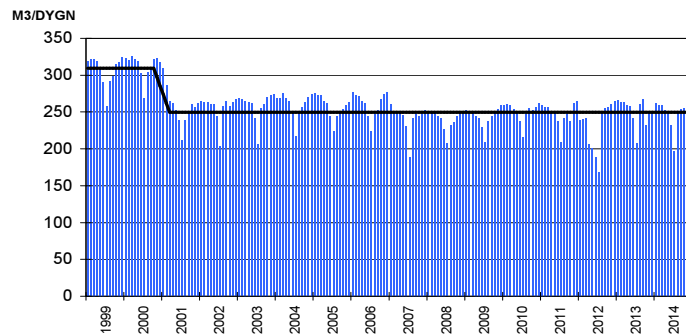
GOTTFRIDSBERG (825 lgh) VATTENBESPARING MONTERAD MÅNAD: nov-00-mar-01
